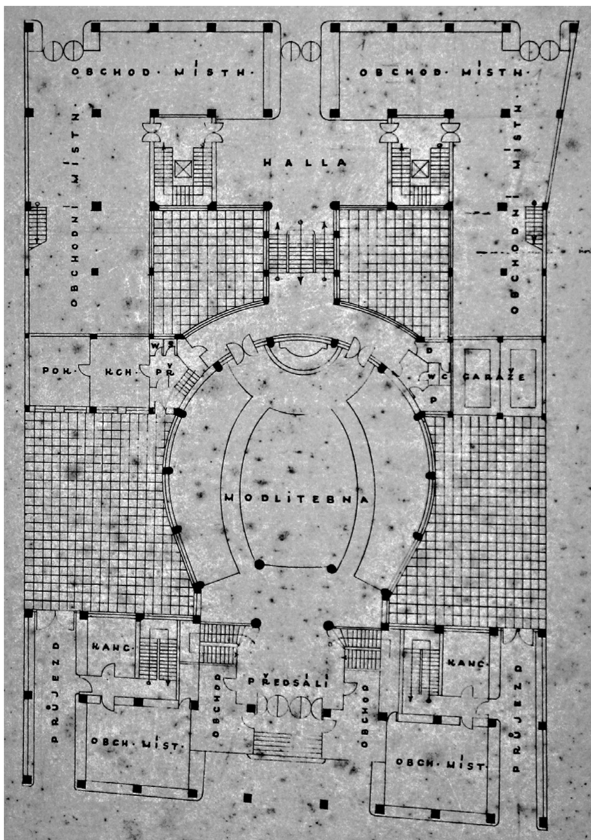
Příloha č. 8. Jaroslav Fišer, půdorys sborových budov (přízemí), duben 1934.
