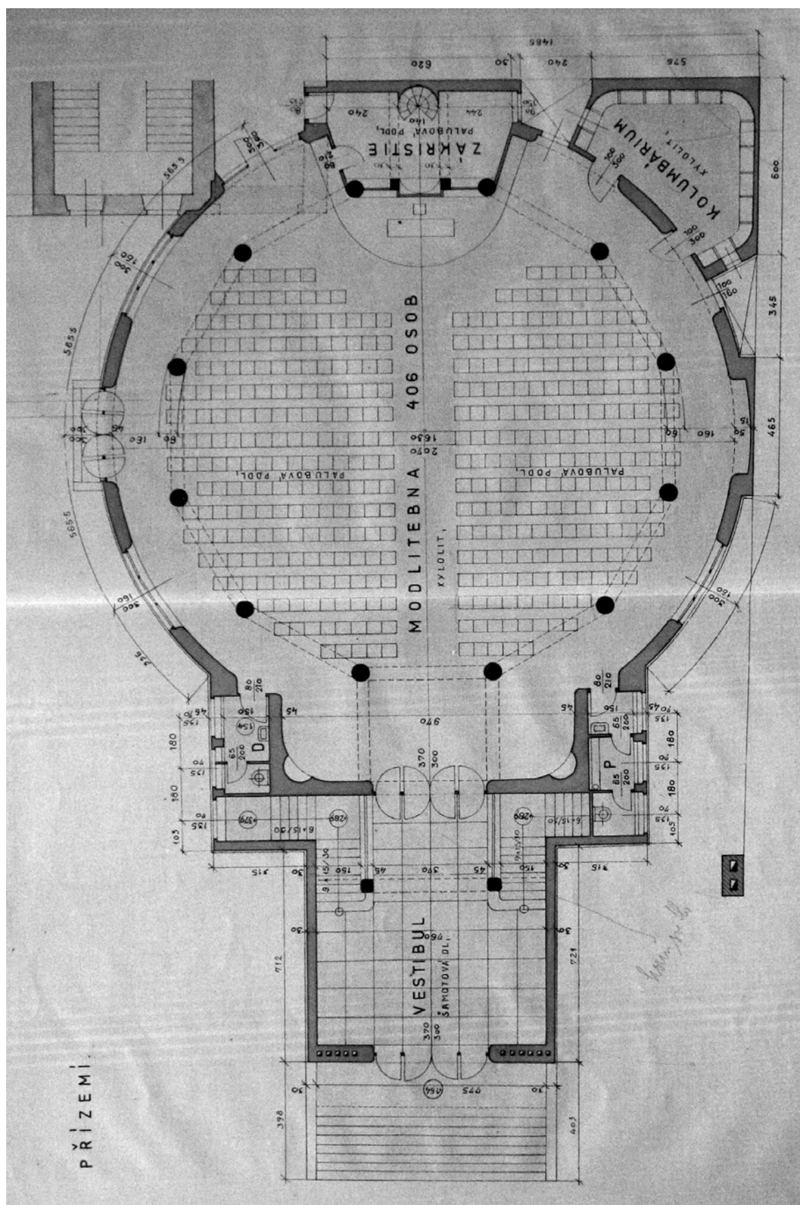
Příloha č. 16. Jaroslav Fišer, půdorys modlitebny (přízemí), srpen 1934.
