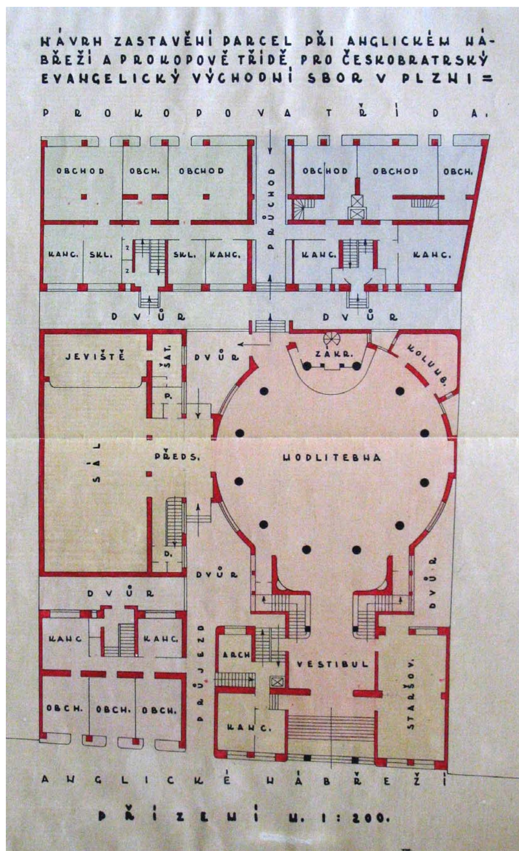
Příloha č. 13. Jaroslav Fišer, půdorys sborových budov, srpen 1934.
