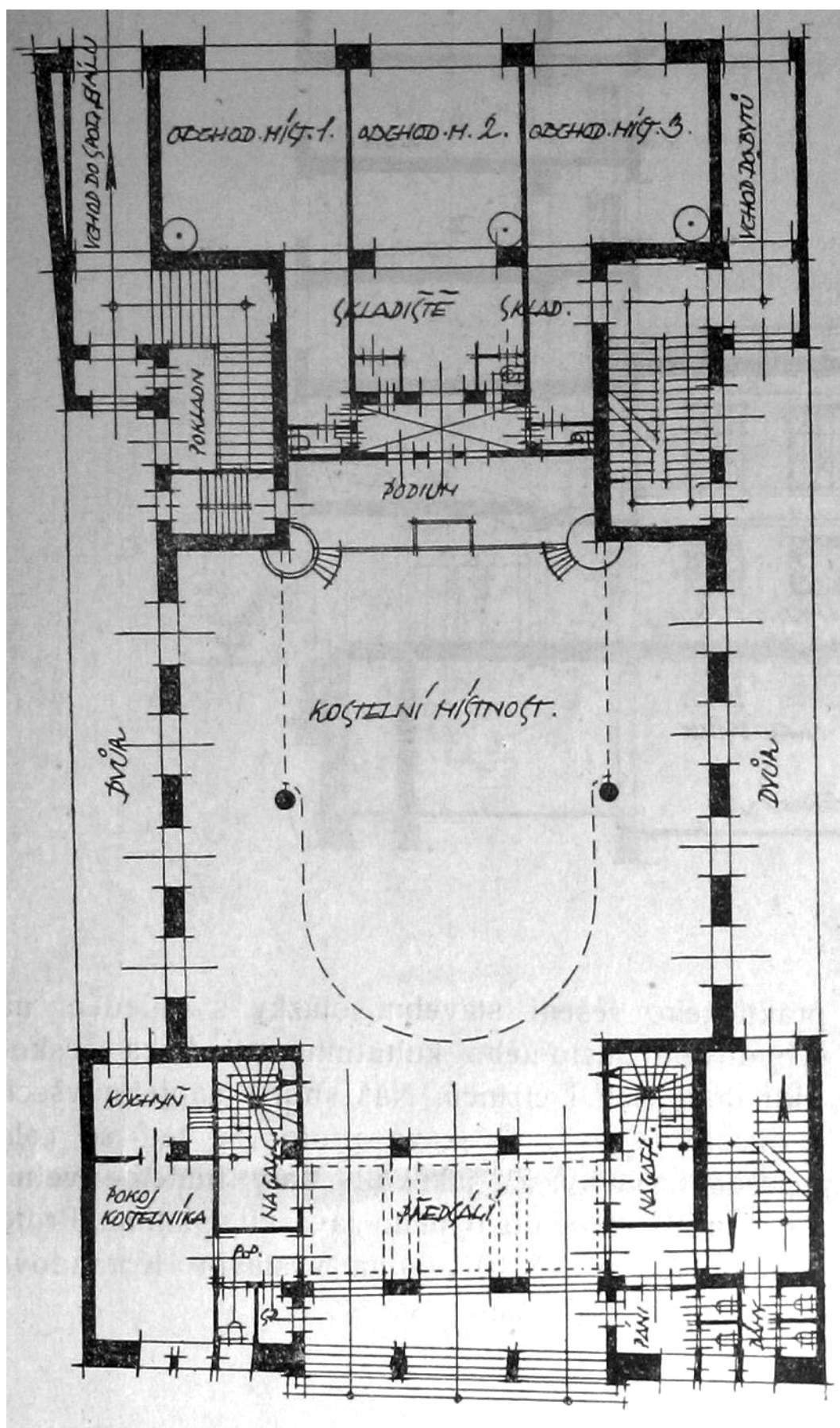
Příloha č. 2. Bohumír Kozák, Korandův dům - půdorys, 1924.
