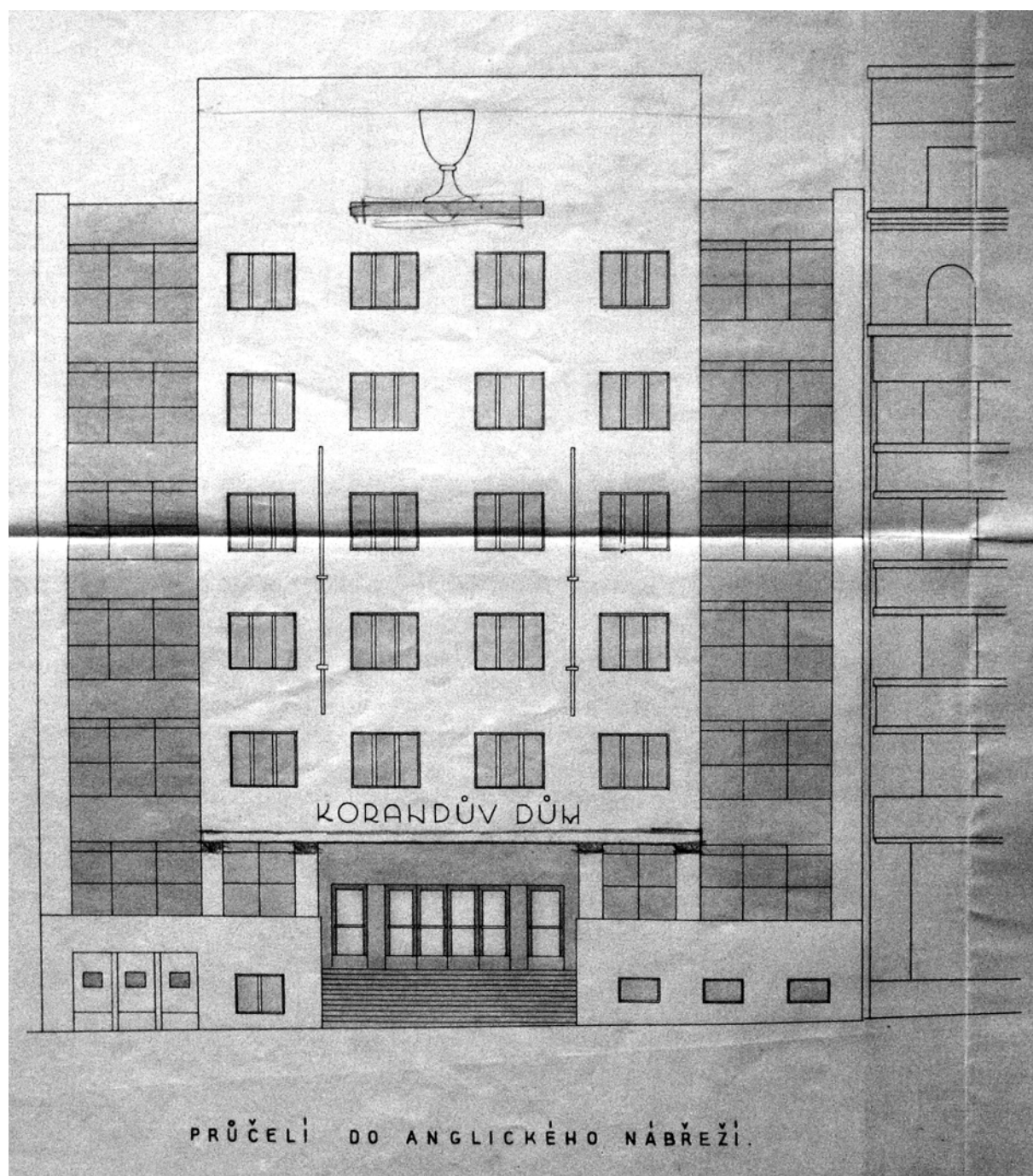
Příloha č. 19. Jaroslav Fišer, pohled z Anglického nábřeží, duben 1935.
